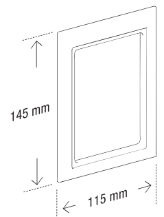
FÜR DEN EINBAU Einbaurahmen mit Putzdeckel Art.-Nr. 24619
